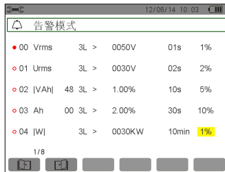
图 5-15 告警模式菜单
