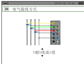
图 4-6 三相 3 线或 4 线连接
