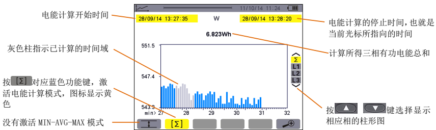
图 10-16 三相有功能量总和和不包括最大、最小、平均值
