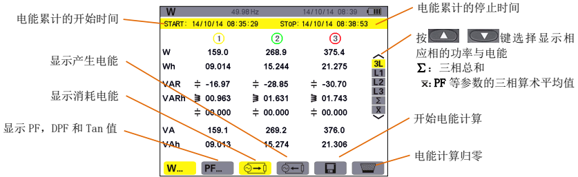
图 11-1 功率和电能屏幕
