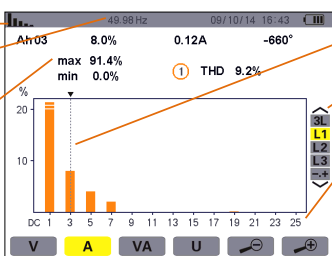
图 7-5 电流谐波 L1 显示
