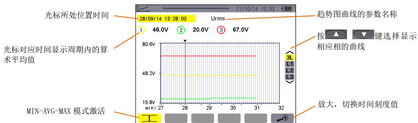
图 10-11 线电压有效值包括最大、最小、平均值
