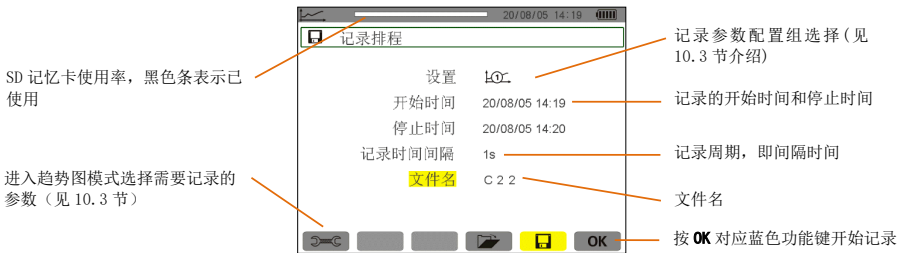
图 10-2 预设记录屏幕图例
