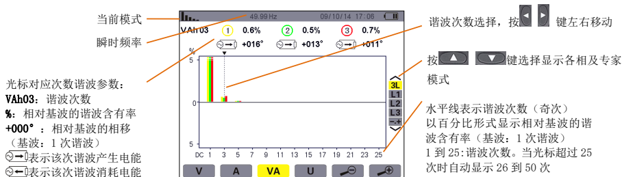
图 7-6 视在功率谐波 3L 显示
