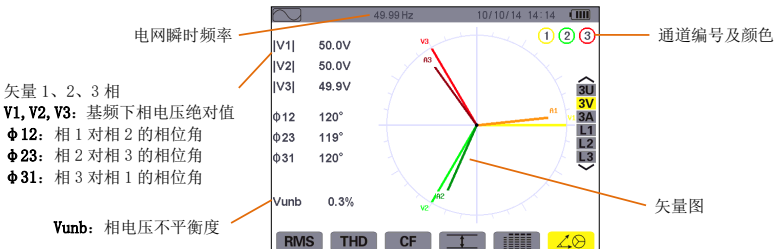
图 8-20 3V 下矢量图示屏幕
