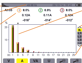
图 7-4 电流谐波 3L 显示
