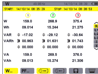
图 11-2 三相(3L)消耗电能的屏幕显示
