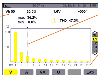
图 7-3 相电压谐波 L1 显示
