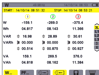
图 11-7 三相(3L)电能产生显示屏幕
