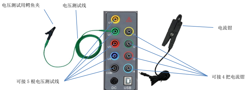
图 4-3 顶端测试连接
