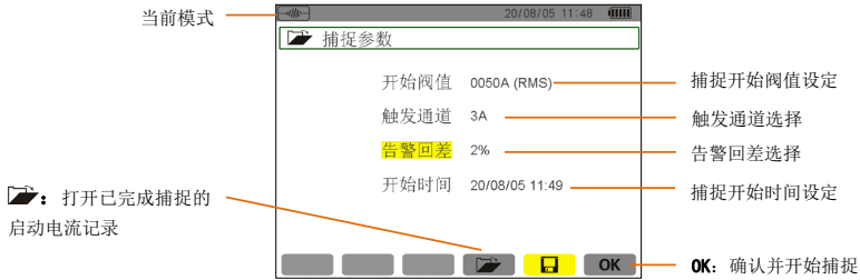
图 6-7 设置启动电流的捕捉排程
