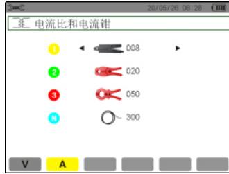
图 5-8 电流钳及变比设置菜单
