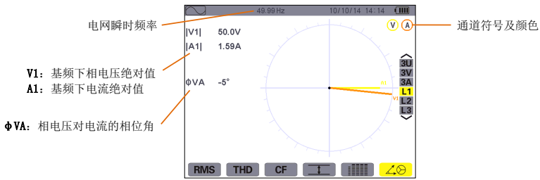
图 8-21 L1 下矢量图显示屏幕
